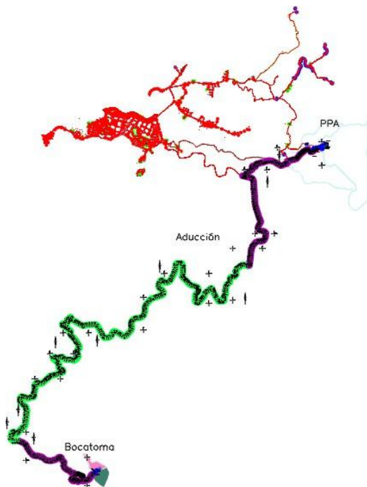
Ilustración 4. trazado nueva aducción
