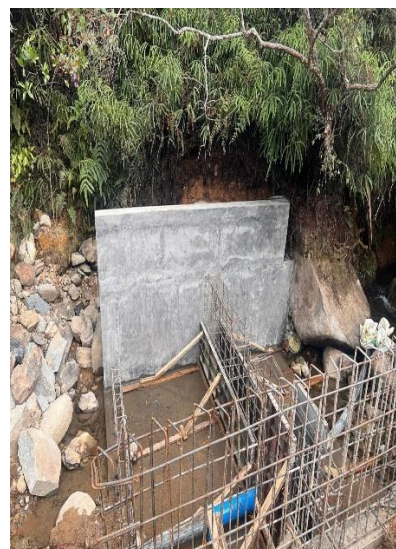
Ilustración 1. Instalación de tubería de la red de aducción y distribución del acueducto
